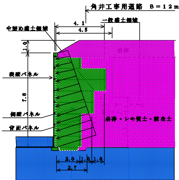
図 - 1 標準断面図
